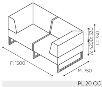
PL 20 CC
