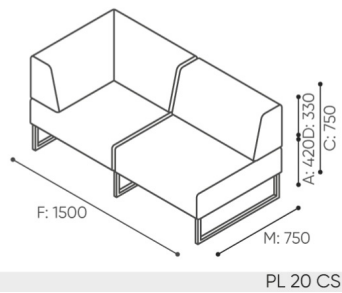
PL 20 CS
